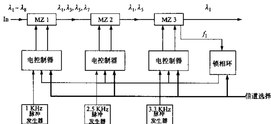
图 10.25 三级可调 MZI 滤波器 (经允许复制于 Wooten et al., © 1993, IEEE)
