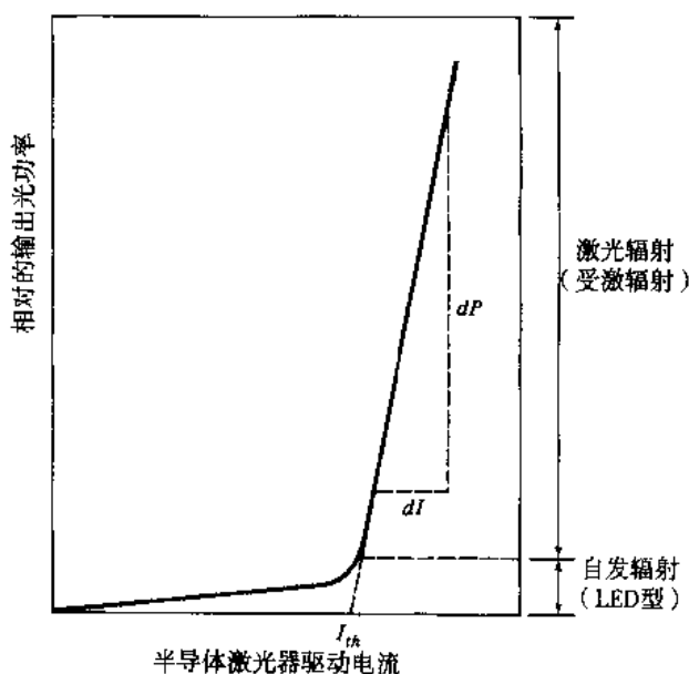
图 4.20 输出光功率与半导体激光器驱动电流之间的关系,在受激辐射阈值点以下,输出光是LED型的自发辐射光
