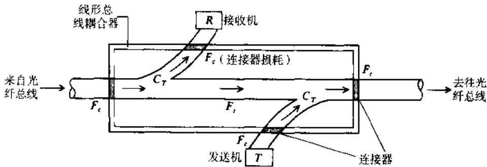
图 12.2 由两个方向耦合器级联而成的无源线形总线耦合器所遇到的损耗
