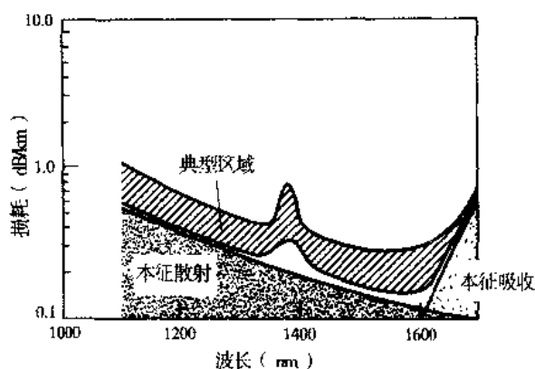
图 3.6 产品级单模光纤的典型损耗谱（经允许复制于 Keck, 16 © 1985, IEEE）
