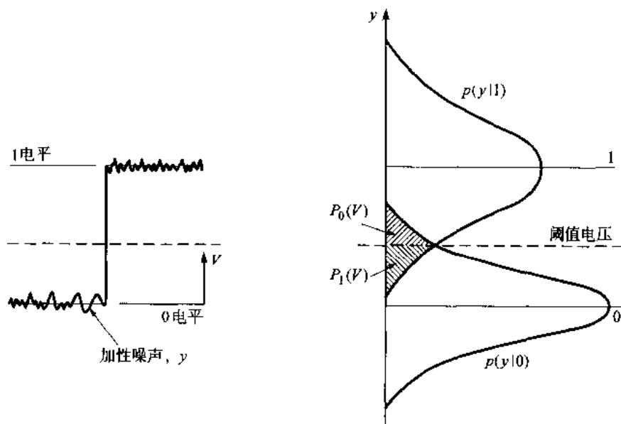
图 7.5 逻辑 0 和逻辑 1 信号脉冲的接收信号概率分布。两种分布的不同宽度是由于各种信号失真所引起的
