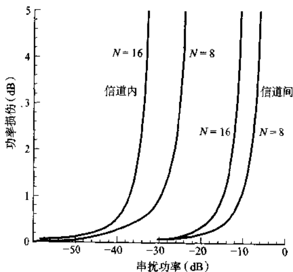
图 12.38 8 和 16 WDM 信道中, 信道内和信道间串扰的功率损伤随单个串扰功率的变化曲线
