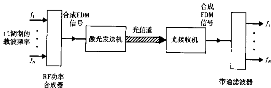
图 9.7 N 个独立的信息承载信号的频分复用标准方法
