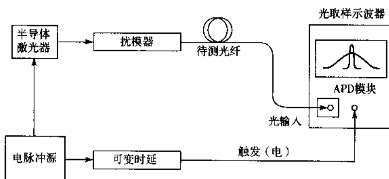
图 13.12 脉冲色散的时域测量法的原理框图
