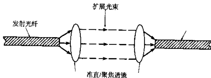
图 5.21 扩展光束光纤连接器的示意图
