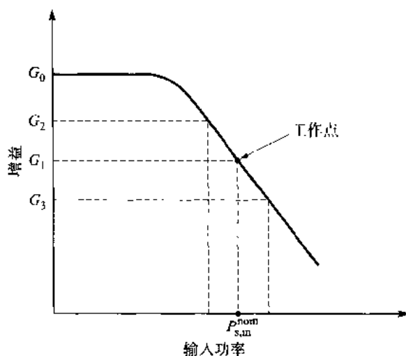
图 11.13 无源信号控制的增益控制方法。在这种方法中,放大器工作在标称输入功率为 P 的饱和区域。输入功率降低会将增益提高到 G_2 , 输入功率增加会使增益降至 G_3
