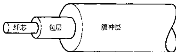
图 2.9 光纤结构示意图。一根折射率为 n_1 圆柱状固体纤, 周围是折射率为 n_2 ( n_2 < n_1 ) 的包层。纤芯和包层封装在一层有弹性的塑料缓冲层中
