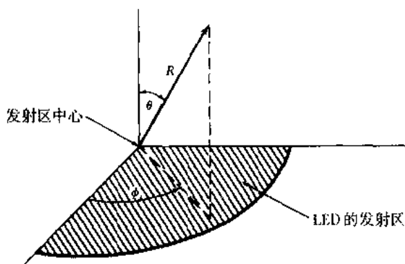
图 5.1 用于表征光源辐射方向图的球面坐标系
