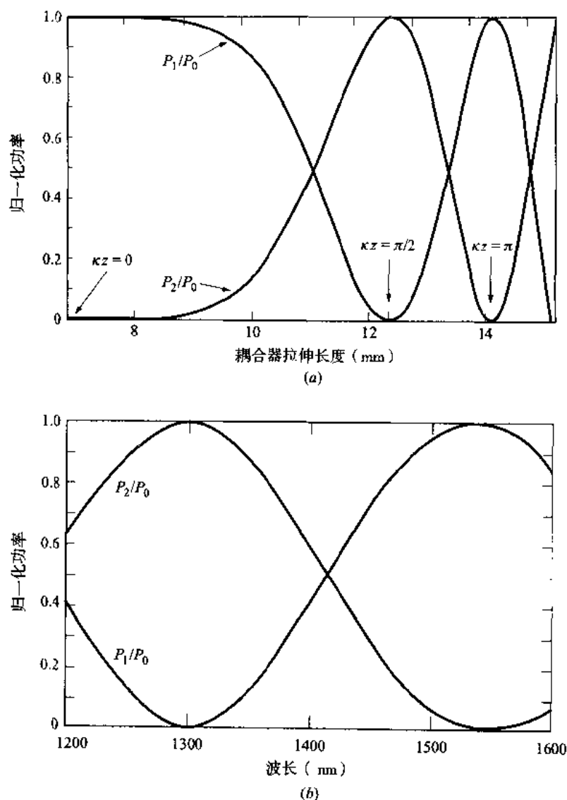
图 10.5 (a) 波长为 1300 nm 的功率 P_0 注入光纤 1 时, 归一化耦合功率 P_2/P_0 和 P_1/P_0 与耦合器长度的函数关系; (b) 在 15 mm 长耦合器中耦合功率与波长的关系 (经允许复制于 Eisemann 和 Weidel, 19 © 1988, IEEE)
