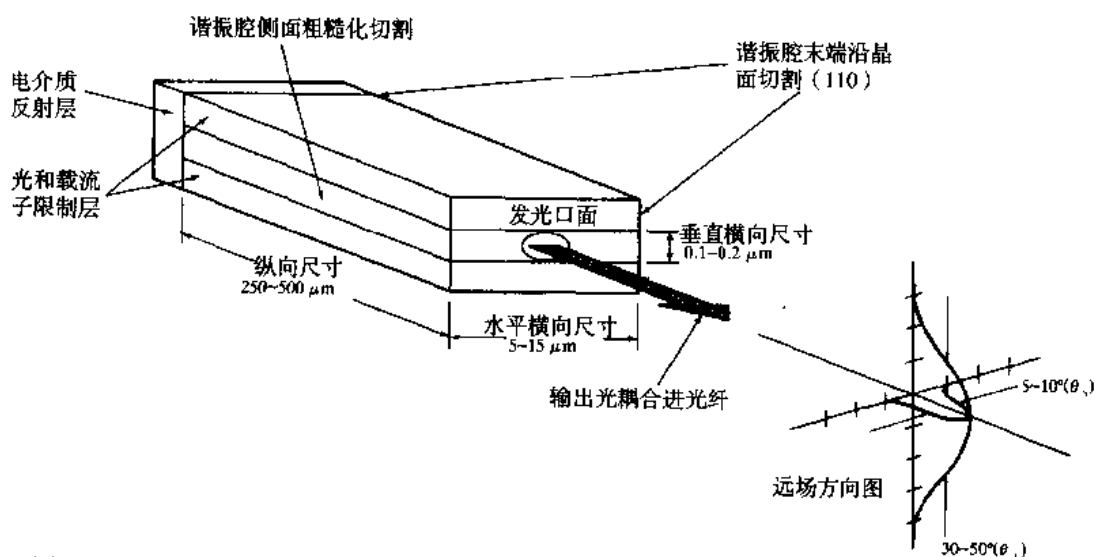
图 4.18 半导体激光器中的法布里-珀罗谐振腔,晶体末端的解理面提供部分反射功能,后端面(未使用)可以涂覆一层电介质反射层以减小腔内的光损耗。注意,尽管在有源区的口面上的激光光斑呈水平椭圆形状,但从激光器发射出的光束形成垂直椭圆形光束
