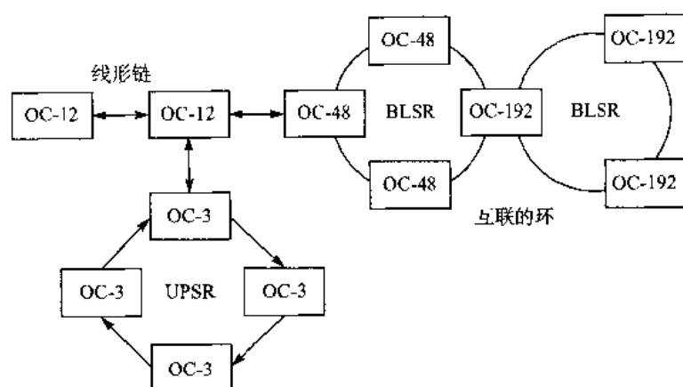
图 12.11 大型 SONET 网络的一般结构，它由线形链以及各种不同类型的环互连组成
