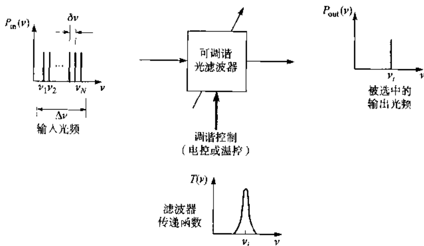
图 10.23 可调谐光滤波器的基本概念
