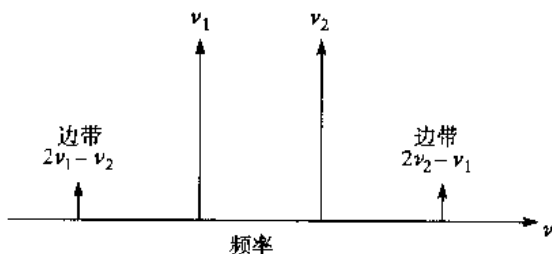
图 12.32 两个频率分别为 \nu_1 和 \nu_2 的光波混频产生两个三阶边带
