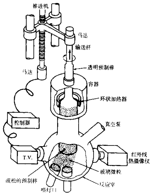
图 2.29 VAD（汽相轴向沉积）方法的设备图（经允许复制于 Izawa 和 Inagaki, 96 © 1980, IEEE）
