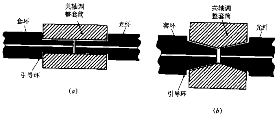
图 5.20 常用光纤连接器的两种对准方案示意图：(a) 直套筒结构；(b) 锥形套筒
