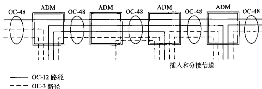
图 12.12 应用于 SONET 的分插复用器的功能概念
