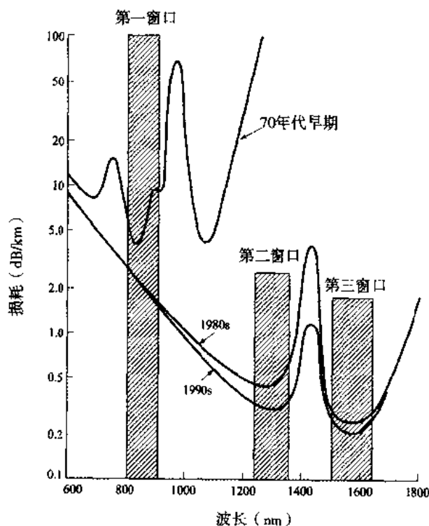
图 1.7 作为波长函数的光纤损耗。早先光纤链路使用 800 nm~900 nm 波段, 将工作波长移至 1310 nm 和 1550 nm 附近的长波长窗口, 可获得更低的损耗
